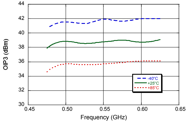
Output IP3_TX1
