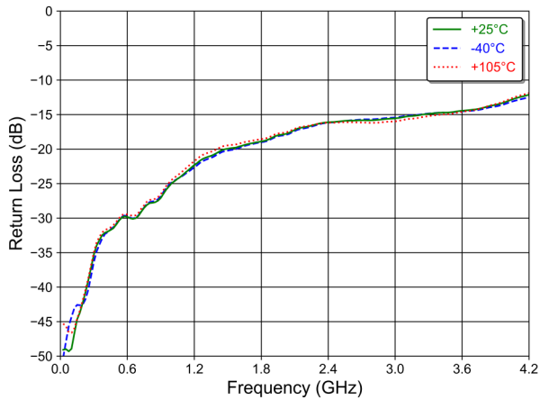
RF1 Return Loss 9 , RFCOM-RF1
