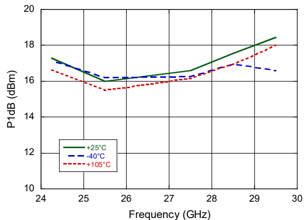
RX P1dB
