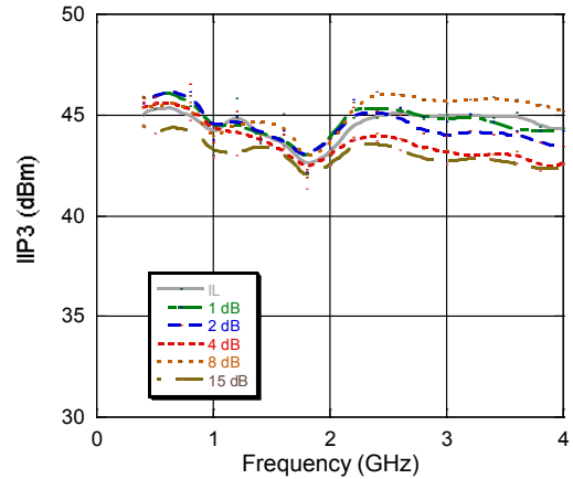
Input IP3
