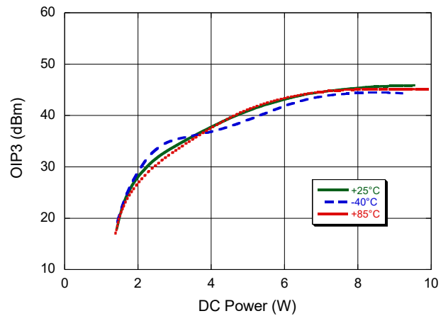
OIP3 @ 19.7 GHz
