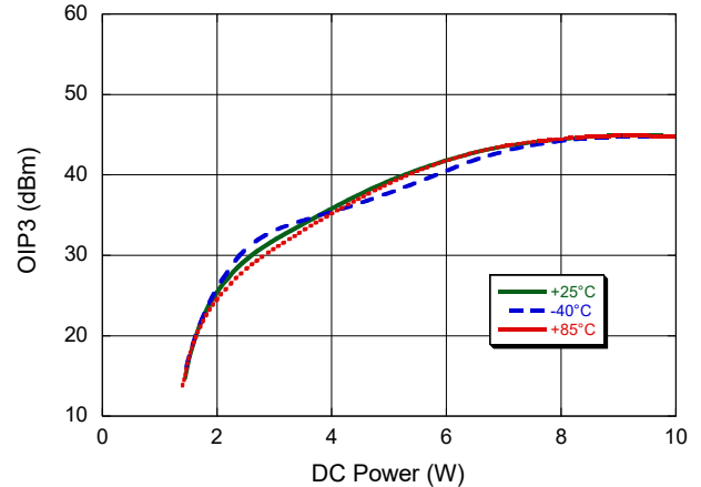
OIP3 @ 19.7 GHz
