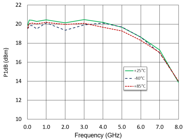
P1dB
